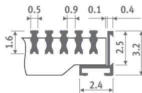
DBR Messingfarben (Nur für Mini Canal)
