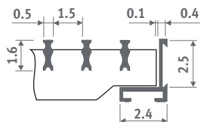
SBR Messingfarben (Nur für Mini Canal)
